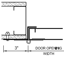
JAMB DETAIL STEEL or WOOD STUD DRYWALL PARTITION
